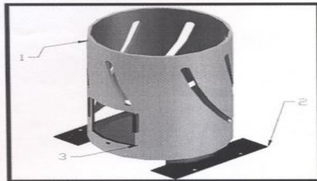
شکل ۲: نقشه ۳ بعدی مخزن شياردار
